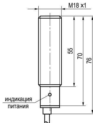
Габаритный чертёж
